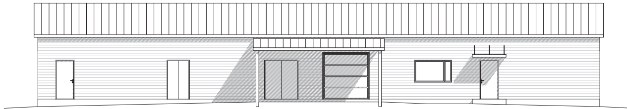
JULKISIVU LÄNTEEN/LOUNAASEEN
