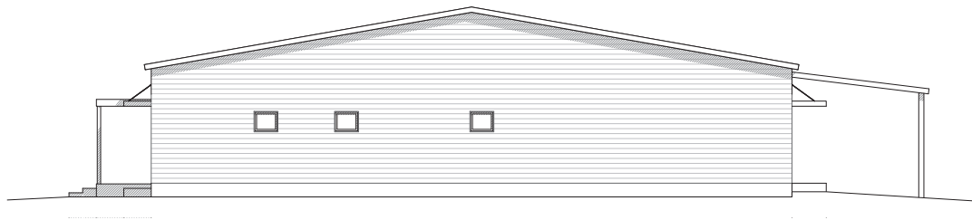
JULKISIVU POHJOISEEN/LUOTEESEEN
