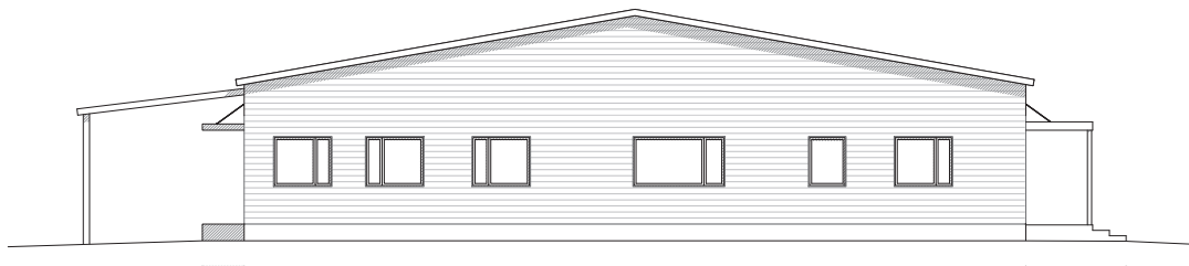
JULKISIVU ETELÄÄN/KAAKKOON
